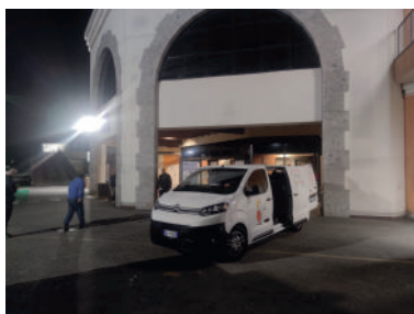
Furgone Citroen Jumpy targato GK779NZ con attrezzatura Mecom PTC Salmon per disotturazioni: motore a benzina, pompa volumetrica, naspo ad alta pressione, radiocomando.
